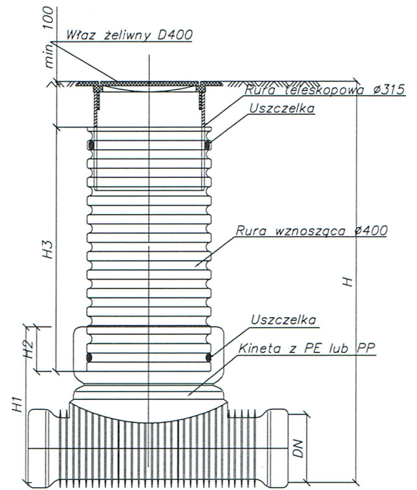
Studzienka kanalizacyjna \varnothing 400 PVC
